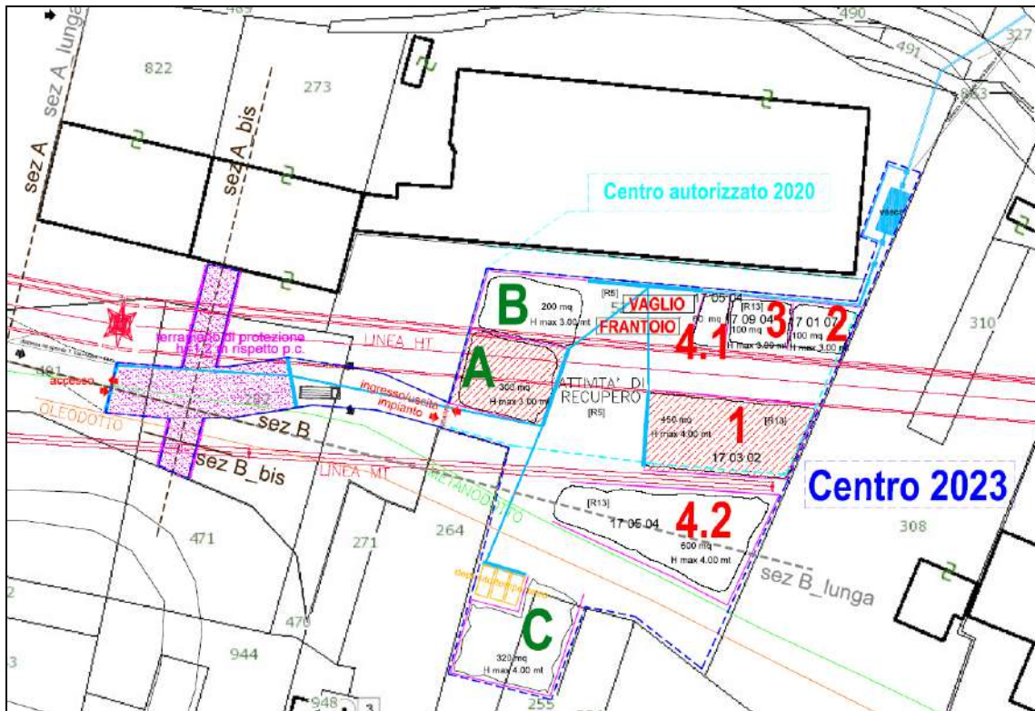
Planimetria dell'impianto
