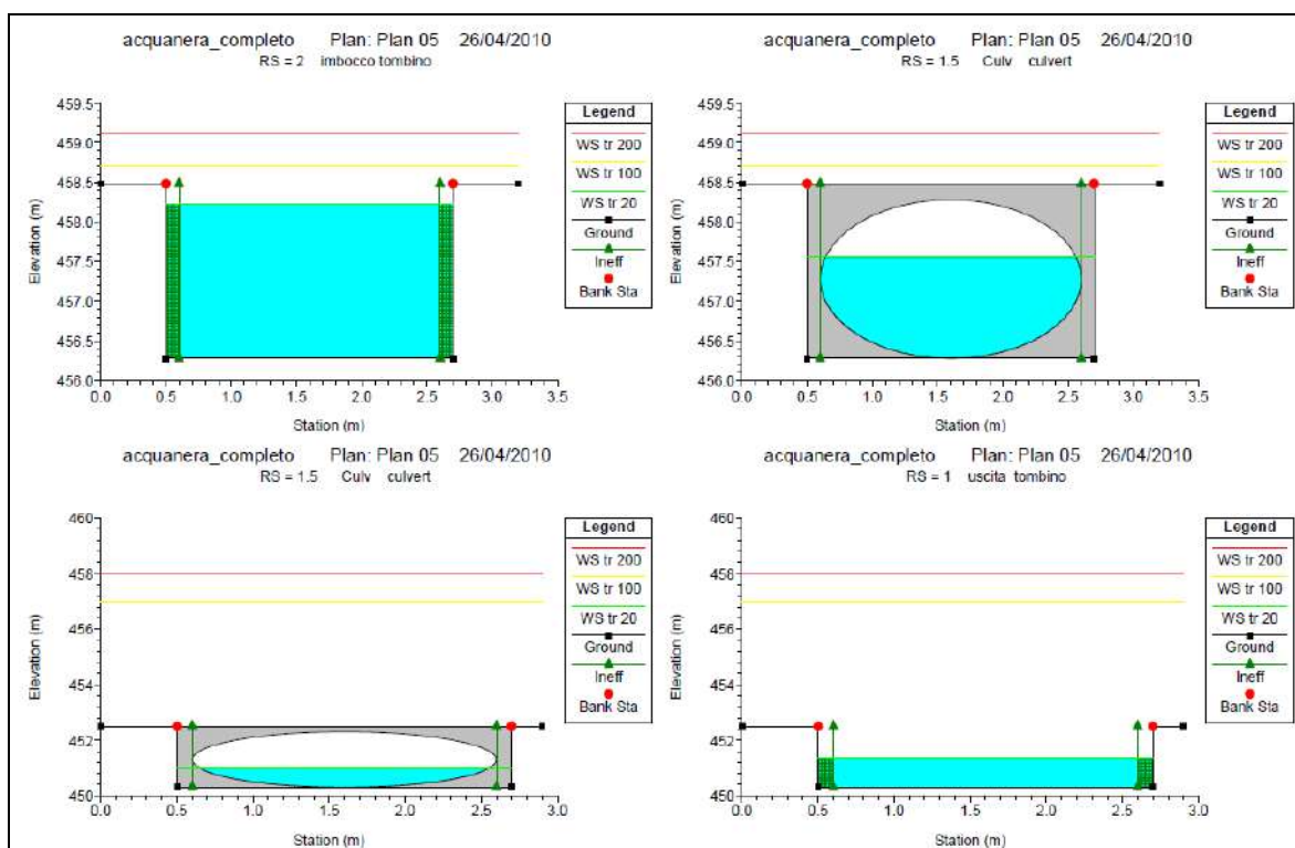
Verifiche idrauliche (RS1=Sez. 55, RS1.5=tratto intubato compreso tra Sez. 55 e Sez. 54, RS2=Sez. 54) Studio di bacino torrente Aqua Nera
